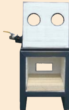
Gasofen SELL mit Schlitz und Zünder ■ Art.-Nr. 11010 (ohne Tür) ■ Art.-Nr. 11012 (mit Tür)
