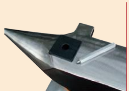
Amboss mit Ambosseinsatz und Durchschläger
