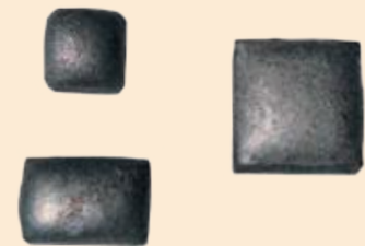
Kornaufschweißplättchen ■ Art.-Nr. 50308 (10 x 10 x 6) ■ Art.-Nr. 50310 (10 x 10 x 8) ■ Art.-Nr. 50320 (10 x 15 x 8) ■ Art.-Nr. 50325 (10 x 15 x 13) ■ Art.-Nr. 50330 (10 x 20 x 13) ■ Art.-Nr. 50340 (15 x 15 x 13)
